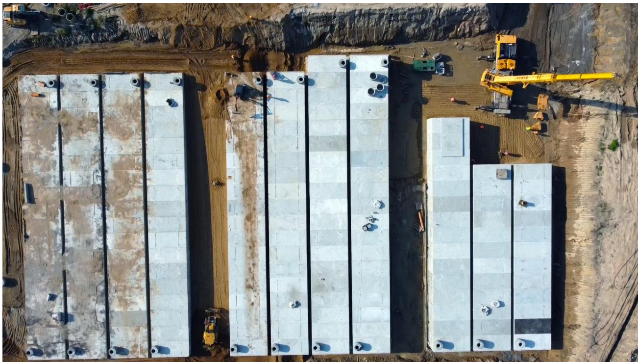
Rysunek 4.3-4: Sienkiewicz MAT-BUD Sp. z o. o. – modułowe zbiorniki typu ZRT – przykłady realizacji
