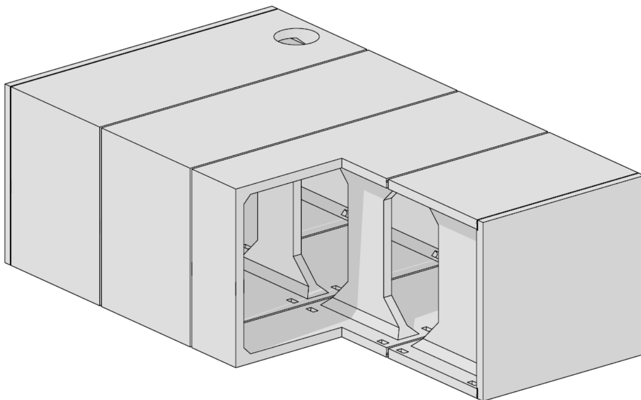
Rysunek 4.5: Sienkiewicz MAT-BUD Sp. z o. o. – wizualizacja modułowego zbiornika typu ZRT
